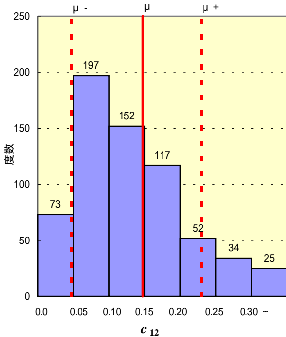
1段タンク型モデル定数
