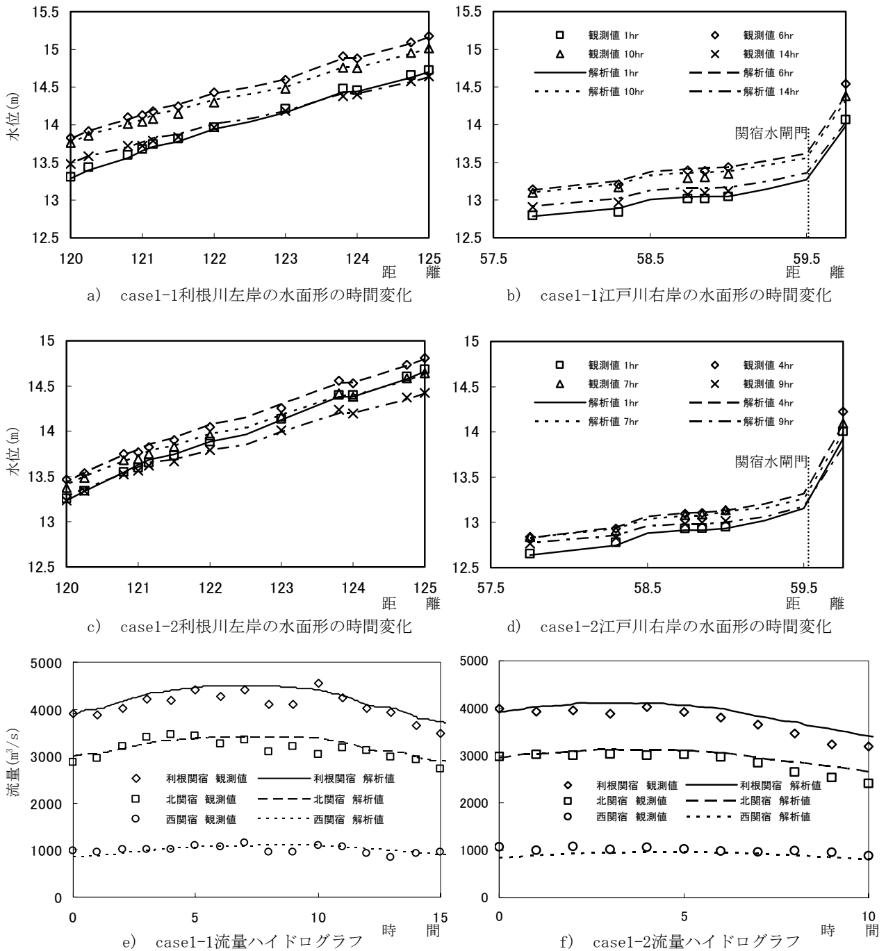
図-5 case1における水面形の時間変化と流量ハイドログラフ
