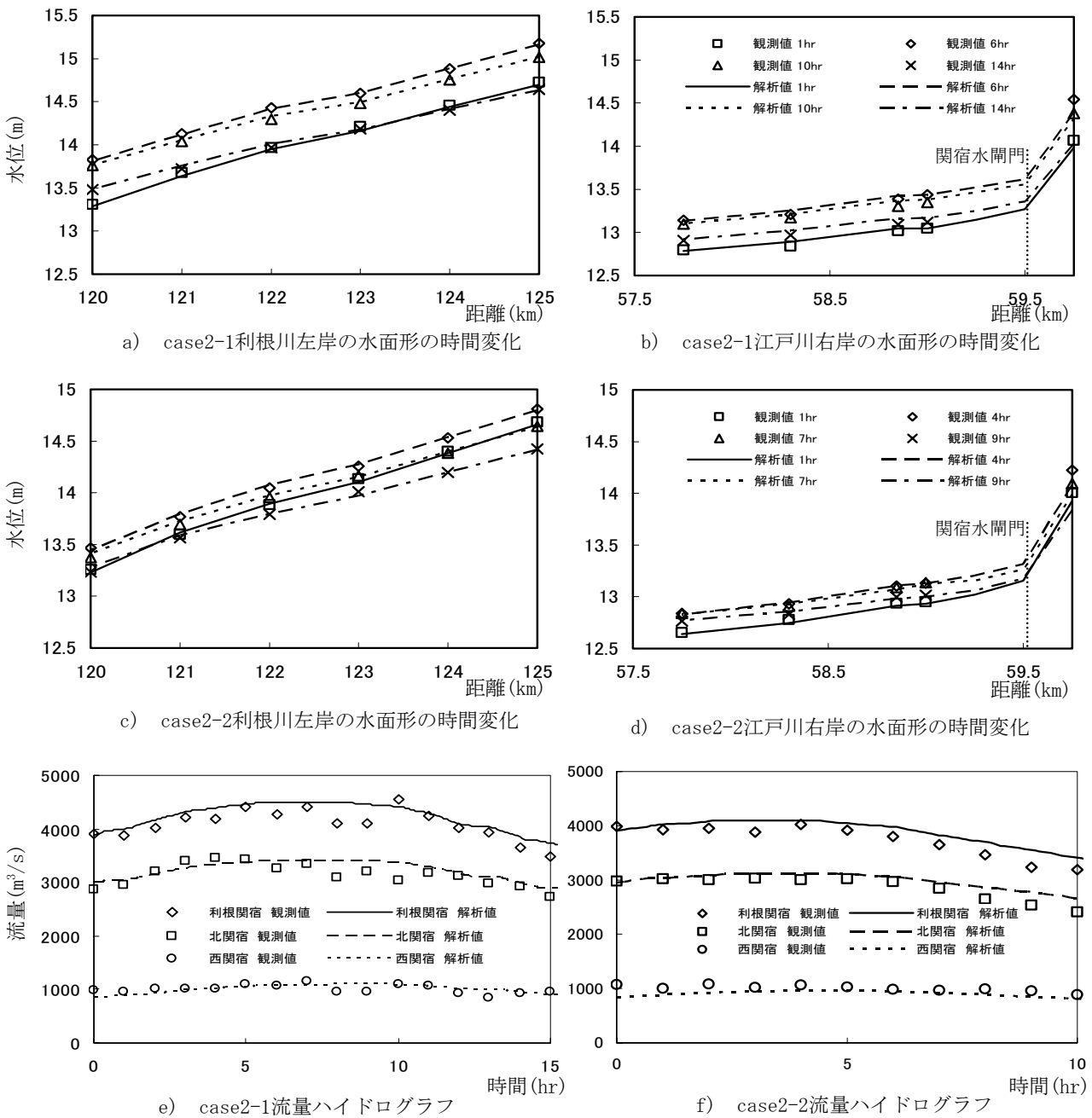
図-6 case2における水面形の時間変化と流量ハイドログラフ
