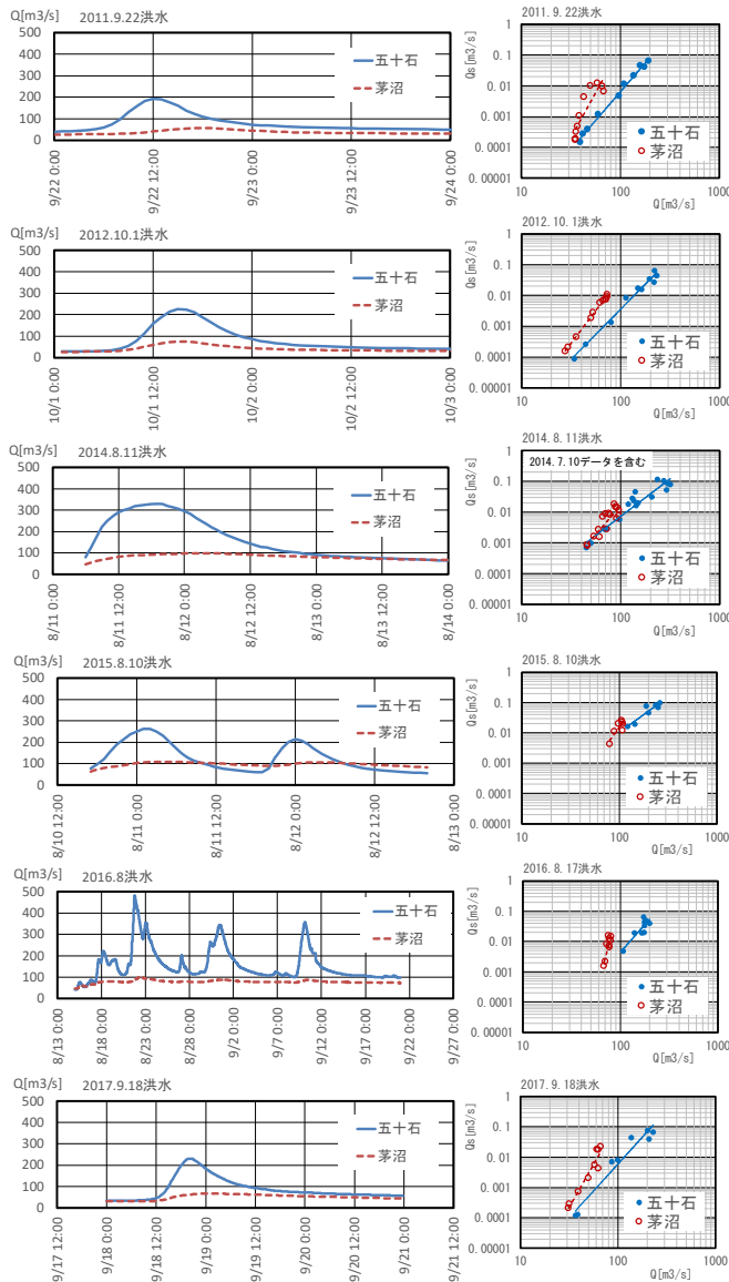
図3 流量・浮遊砂量観測結果
