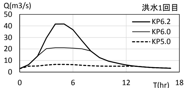
図5 河道流量算定結果 (KP6.2: 旧川流入前, KP6.0 旧川流入直後, KP5.0 旧川復元区間)
