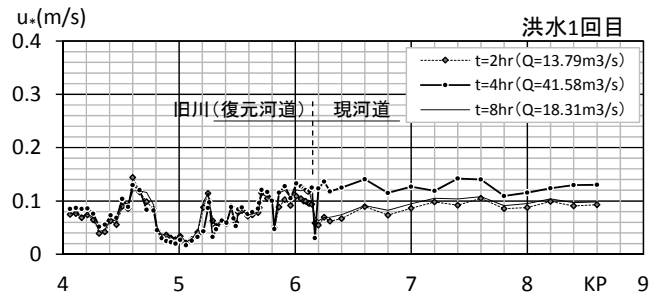
図6 摩擦速度縦断面図
