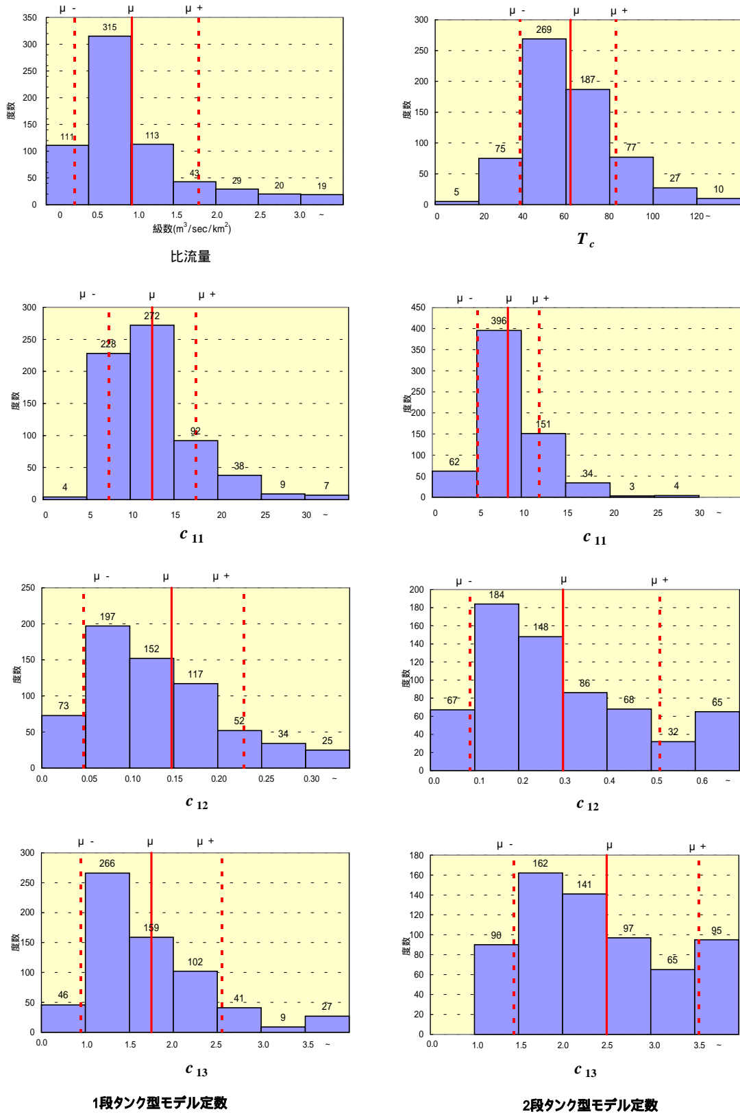
図3.16 全水系における1段・2段タンク型モデル定数の比較
