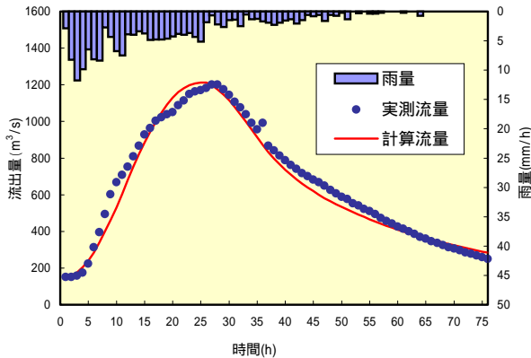
図2.15 渚滑川(上渚滑, 流域面積: 1050.60km 2 ) 2001年9月10日~9月13日洪水
