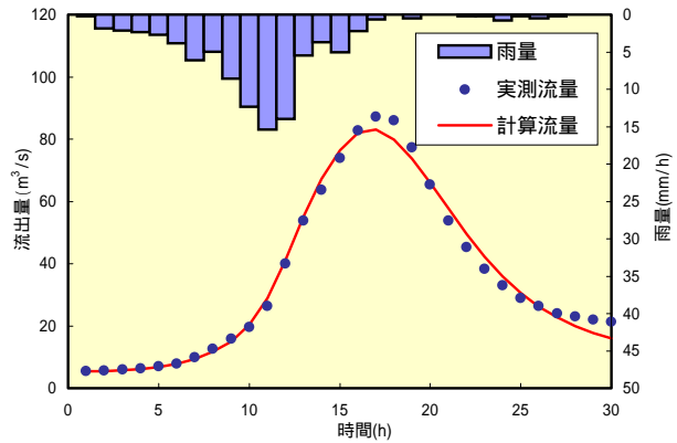
図2.14 美幌川(美幌橋, 流域面積: 199.30km 2 ) 1998年9月16日~9月17日洪水
