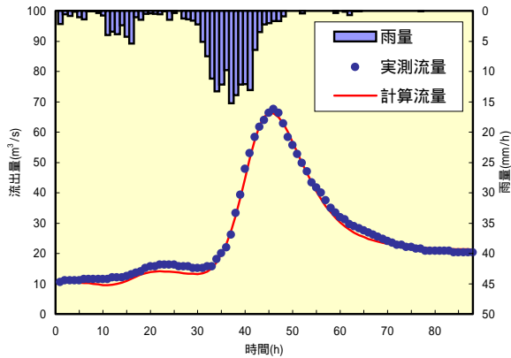
図2.13 釧路川(弟子屈, 流域面積: 127.80km 2 ) 1992年9月10日~9月13日洪水
