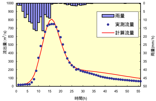
図2.16 後志利別川(今金, 流域面積: 361.40km 2 ) 1986年9月21日~9月23日洪水
